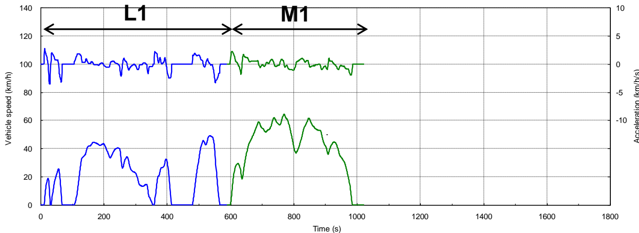
Class 1 WLTC ver.2.0
