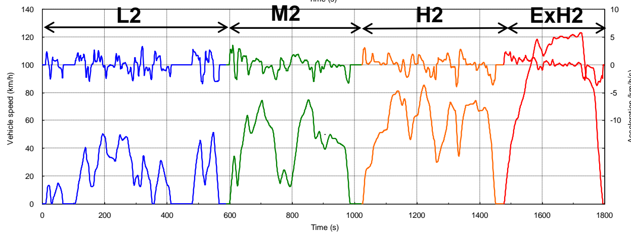
Class 2 WLTC ver.2.0
